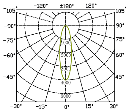
Curva de distribución de la luz.
